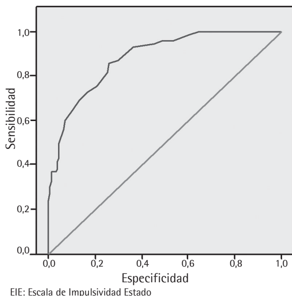
Figura 1 Curva ROC de la EIE: Puntuación total
